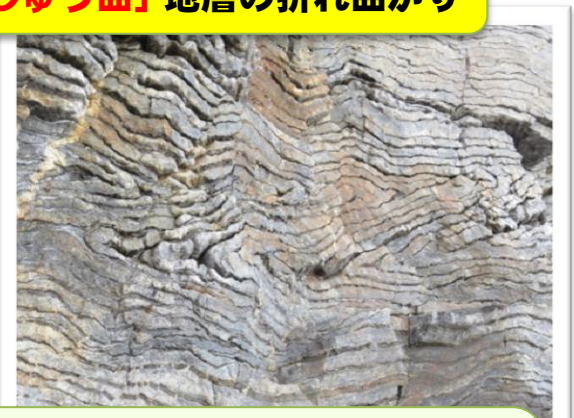
「日見崎のしゅう曲」地層の折れ曲がり
